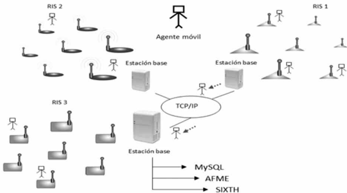
Figura 3. Arquitectura mejorada de interconexión de diferentes RIS heterogéneas usando el sistema embebido como estación base para cada una de las redes
