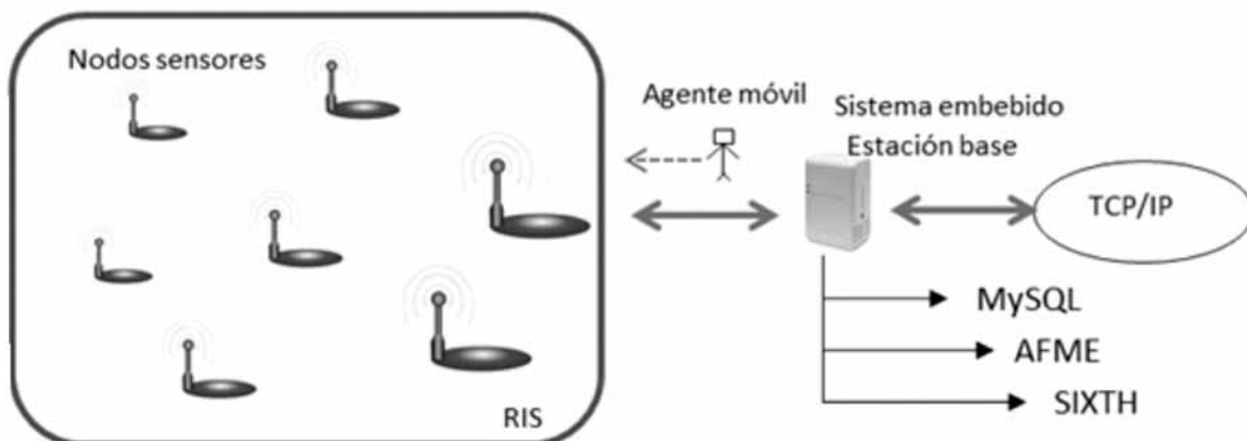
Figura 1. Arquitectura inicial de la solución propuesta, usando el sistema embebido y agentes móviles inteligentes para reprogramar la RIS
