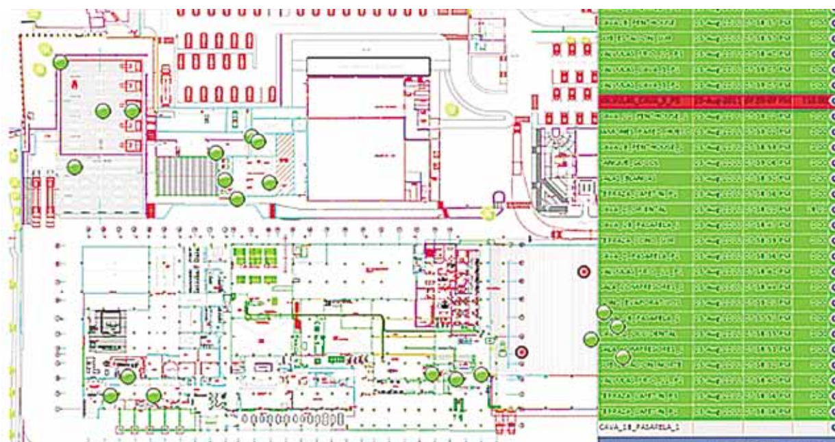
Figura 2. Vista de la planta de producción de alimentos cárnicos y la aplicación donde se aprecia la ubicación de algunos sensores (círculo verde)
