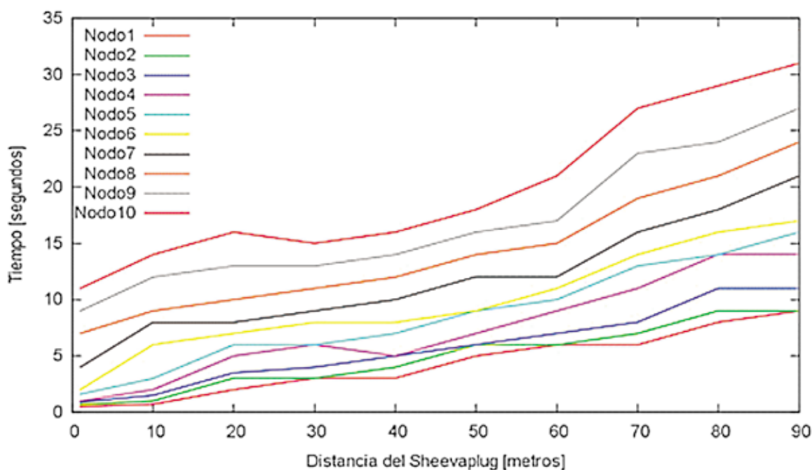
Figura 4. Tiempo de convergencia en la reconfiguración autónoma de un parámetro contra distancia
